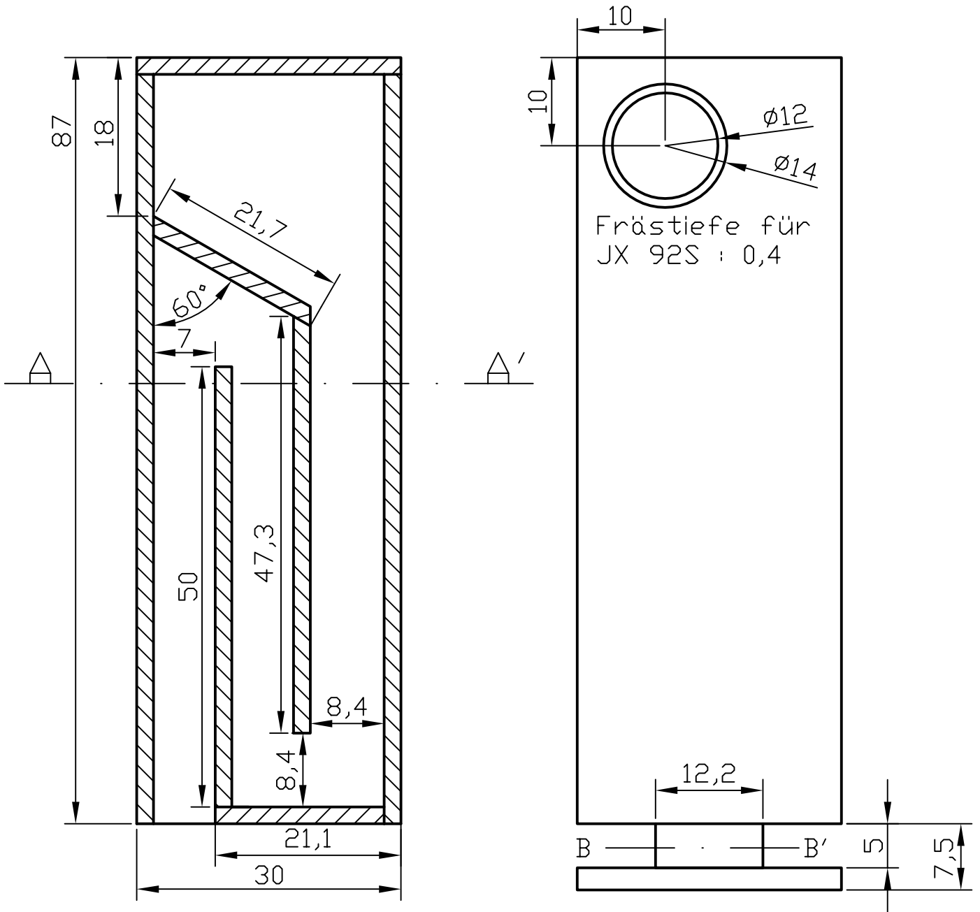
Schnitt A-A'
