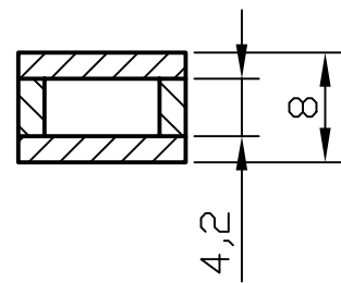
Schnitt B-B'
