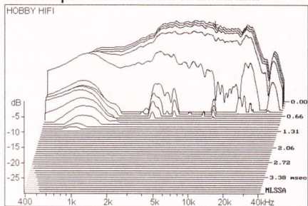
Sehr schnelles und gleichmäßiges Ausschwingen, erkennbare Resonanzfrequenz um 1 kHz.
