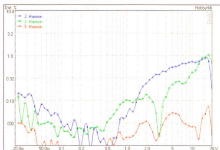
Erst bei größerer Lautstärke ansteigende, selbst bei 20 Volt (entsprechend 110 dB bei 2 kHz) noch sehr moderate Verzerrungen.
