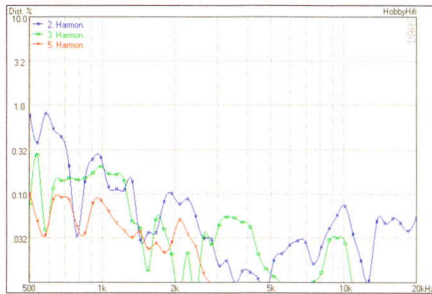
Extrem geringe Verzerrungen, auch unter 1 kHz vorzügliches Klirrvverhalten.
