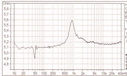
Bei starker vertikaler Spreizung ist die Resonanzfrequenz bei 900 Hertz bestens erkennbar.
