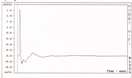
Optimales Ein- und ganz minimal verzögertes Ausschwingen.
