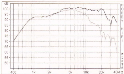
Ab 4 kHz hervorragend linear und ausgewogen, phänomenaler Wirkungsgrad.
